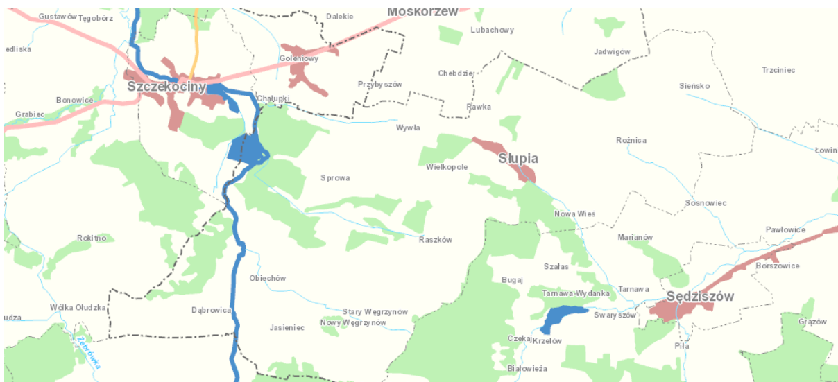
Mapa 3 Zagrożenie powodziowe na terenie Gminy Słupia
